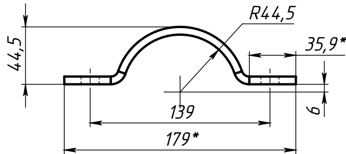
Поз.4 (Полухомут)
