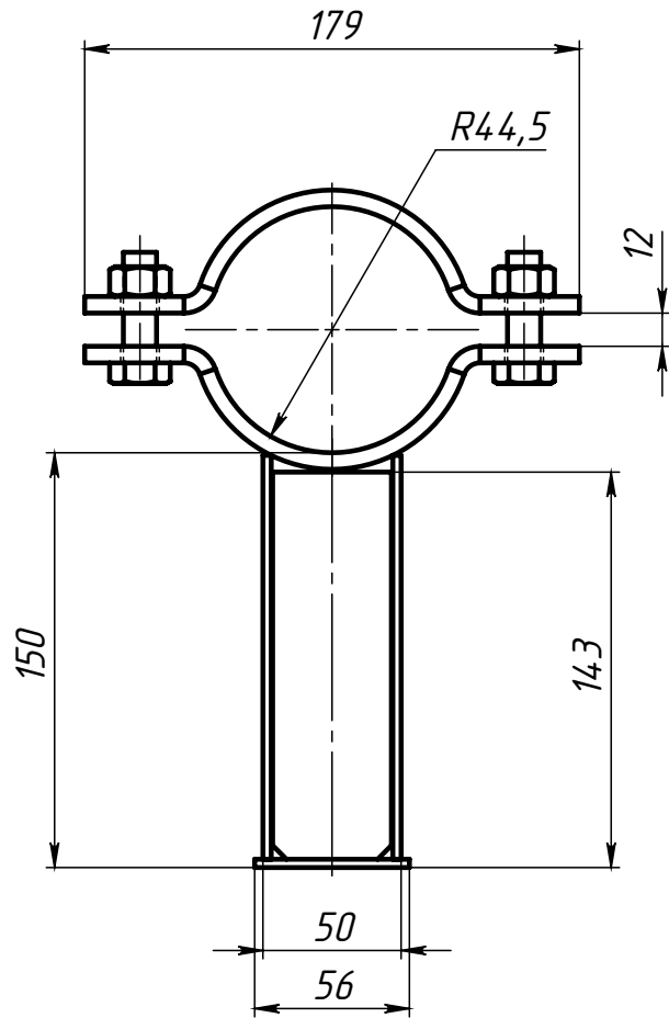
Поз.4 (Полухомут)
